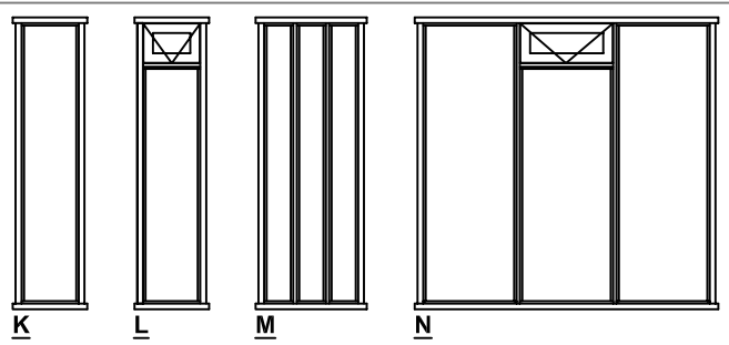
kloosterkozijnen
