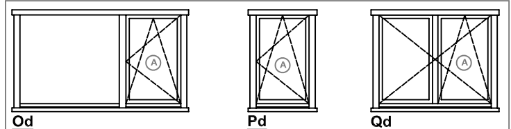
draaivalraamkozijnen
